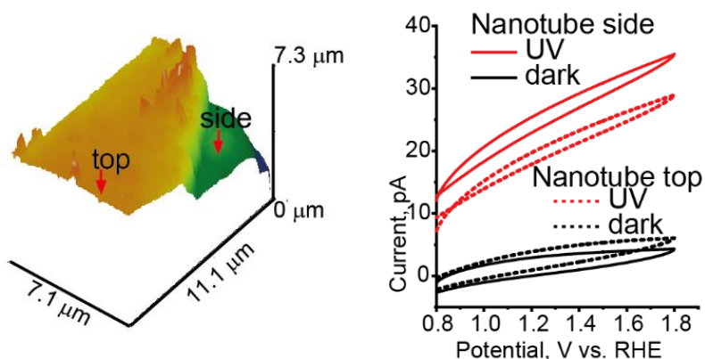
図3 TiO 2 ナノチューブアレイの三次元凹凸像と局所的な光電流応答。 チューブの最上部と側面とで光電流値に大きな差は認められなかった。
